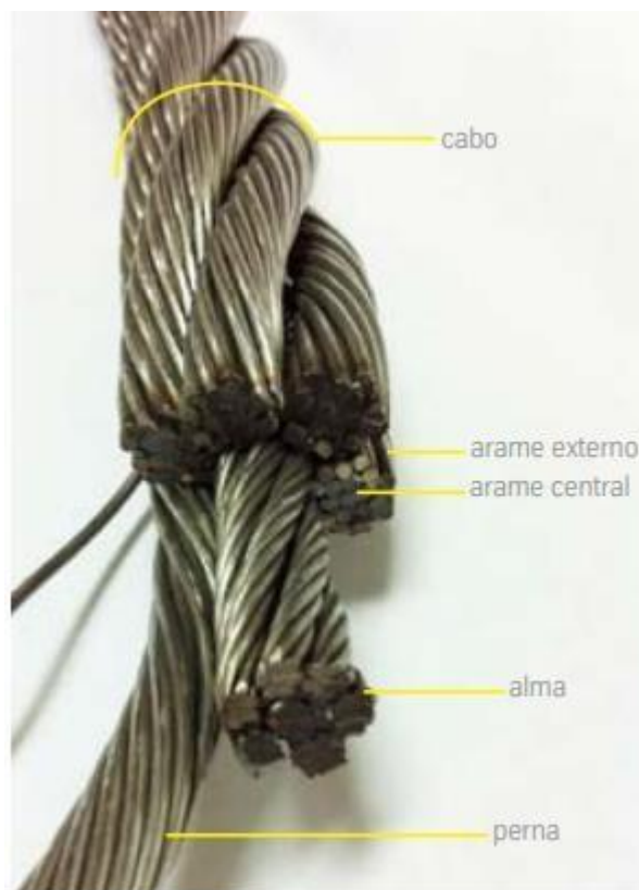
Composição do cabo de tração
