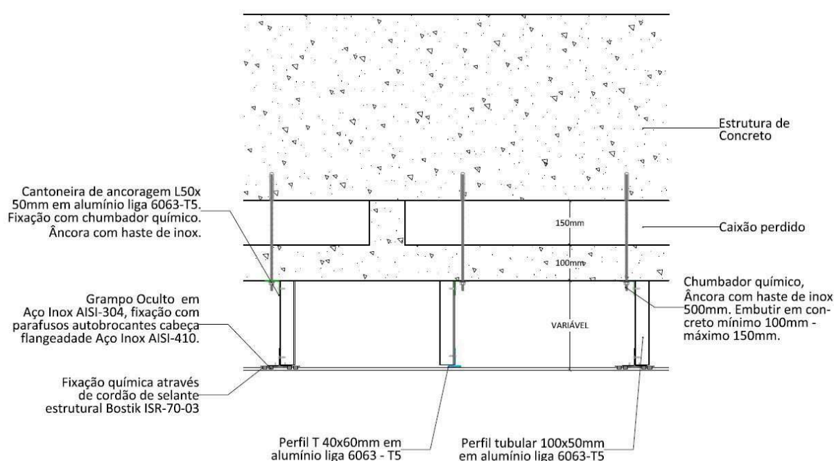
DET.1 - ANCORAGEM NAS PRUMADAS FRONTAIS E POSTERIORES A e B
