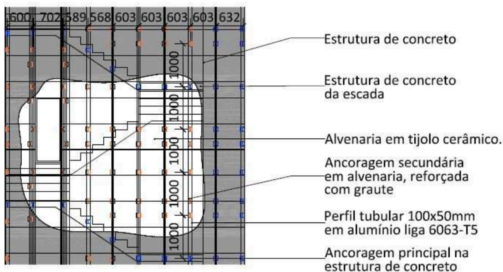
DET. 4 - FACHADA VENTILADA (ANCORAGEM NAS PRUMADAS 1A / 4B) ESCALA 1:50
