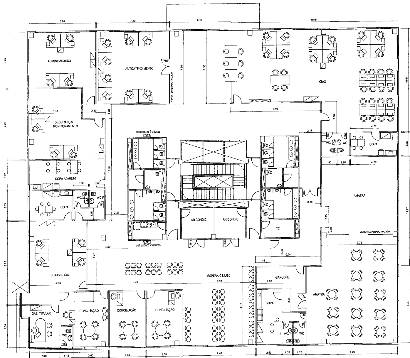
PANAMÉRICA PARK - BLOCO 02 - 2º PAVIMENTO
