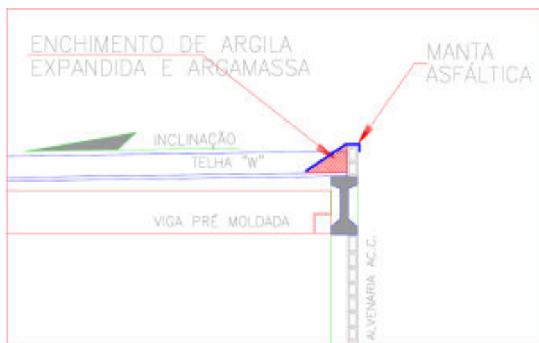
Figura-5: Aplicação de argila e manta asfáltica na lateral do prédio.
