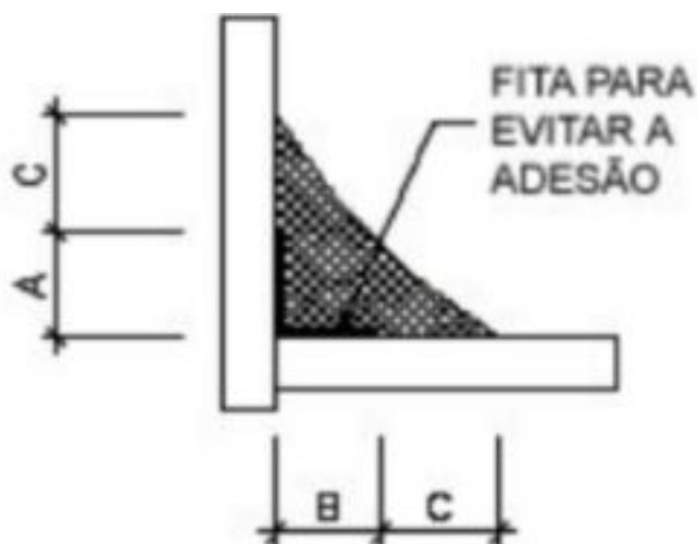
Figura-4: Detalhe de execução da aplicação de silicone nas esquadrias.
