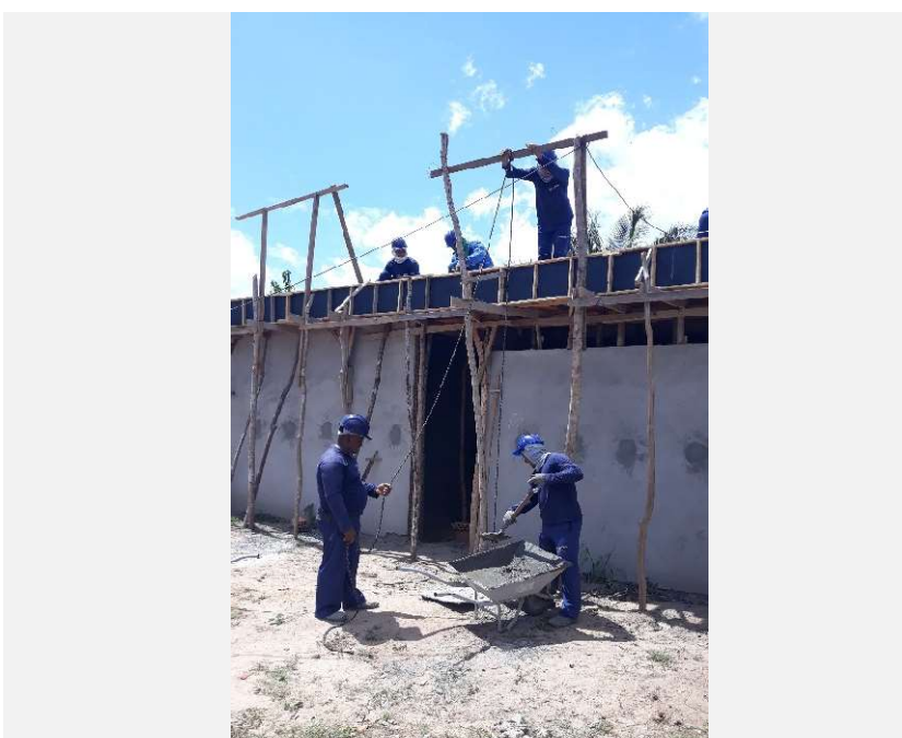
Execução de concretagem de lajes.
