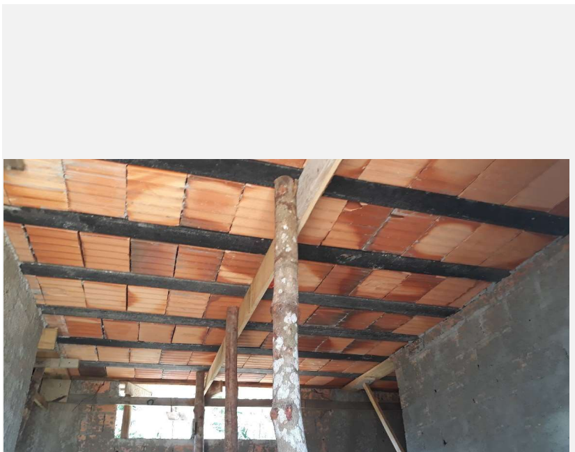
Execução de concretagem de lajes.
