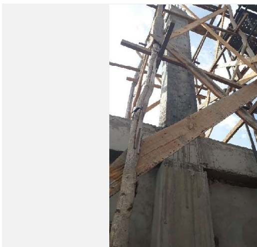
Execução de pilares.
