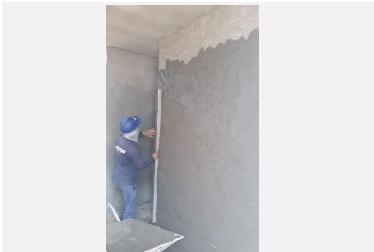
Execução de emboço interno.
