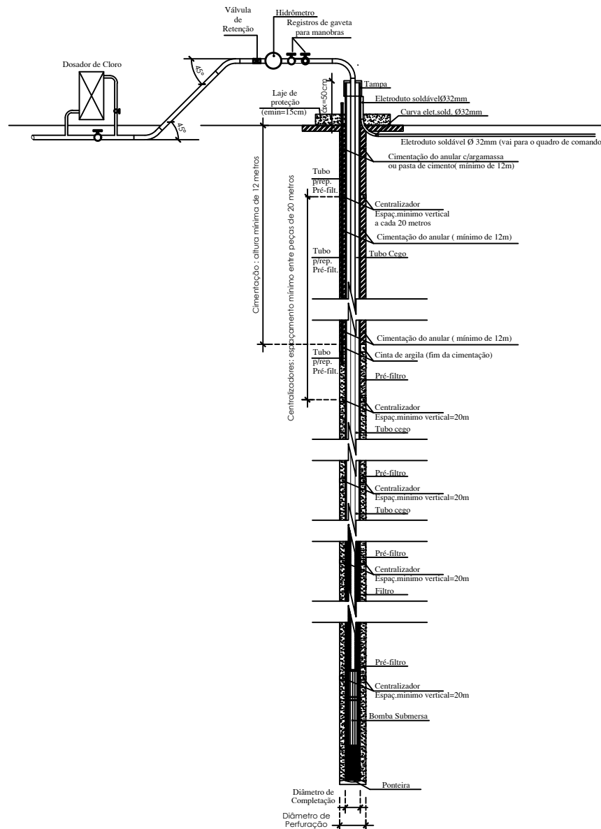
PERFIL SEMI ARTESIANO Sem Escala
