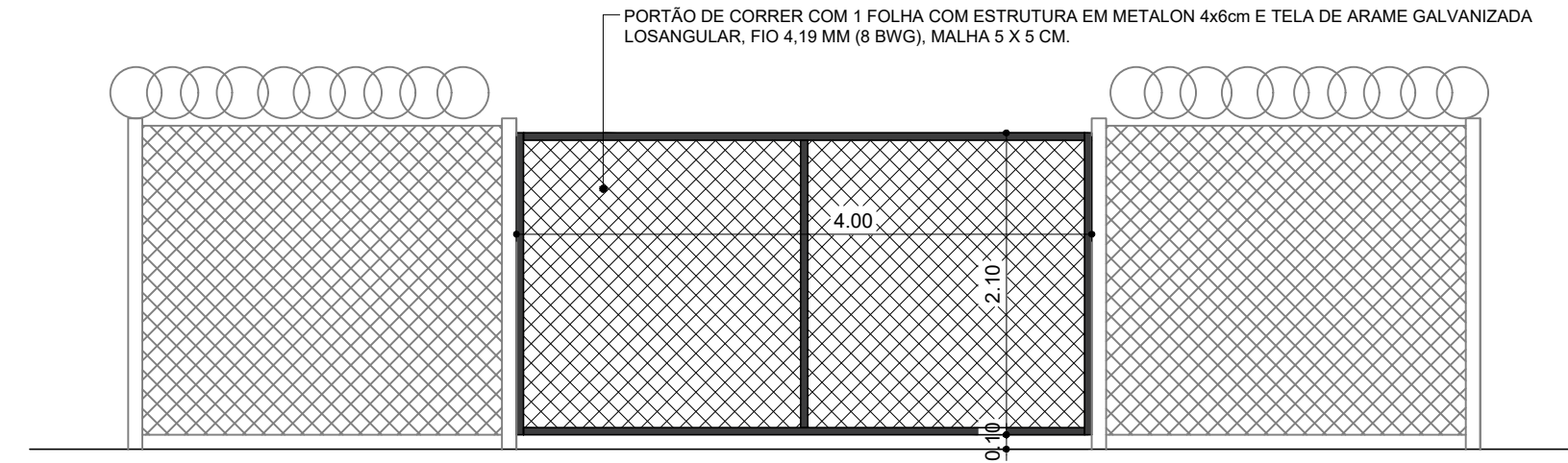
PORTÃO ESCALA 1/50
