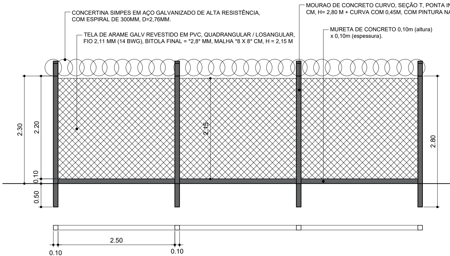
FECHAMENTO ESCALA 1/50
