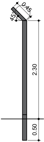
VISTA LATERAL ESCALA 1/50
