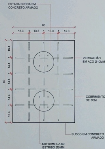
PLANTA DE FUNDAÇÃO ESCALA 1/10
