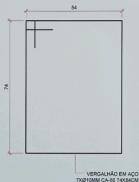
PLANTA DE FERRAGENS ESCALA 1/10
