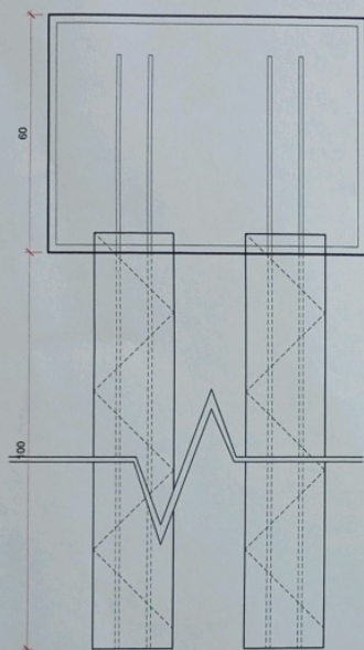
CORTE ESCALA 1/10
