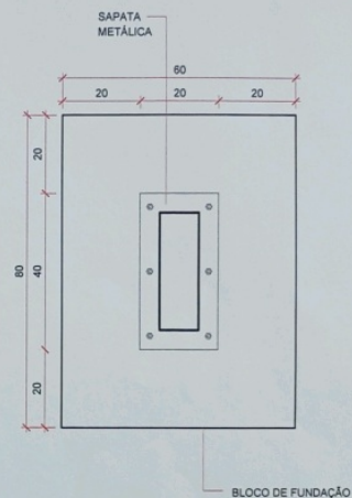
LOCAÇÃO BLOCO FUNDAÇÃO ESCALA 1/10
