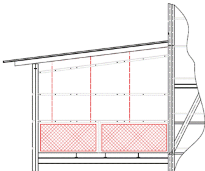
Figura 2 - Tela galvanizada malha 2x2.
