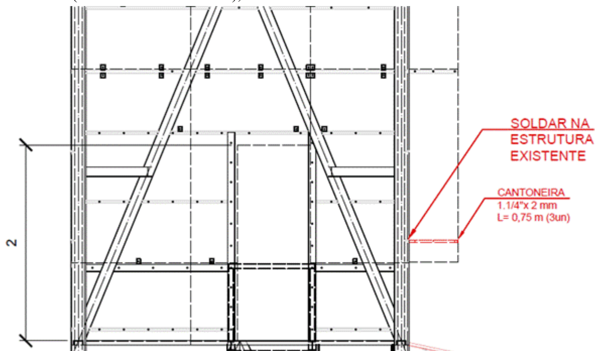
Figura 1 - Local para instalação do suporte de fixação.
