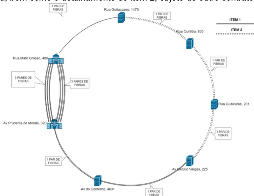
Figura 1: Topologia
